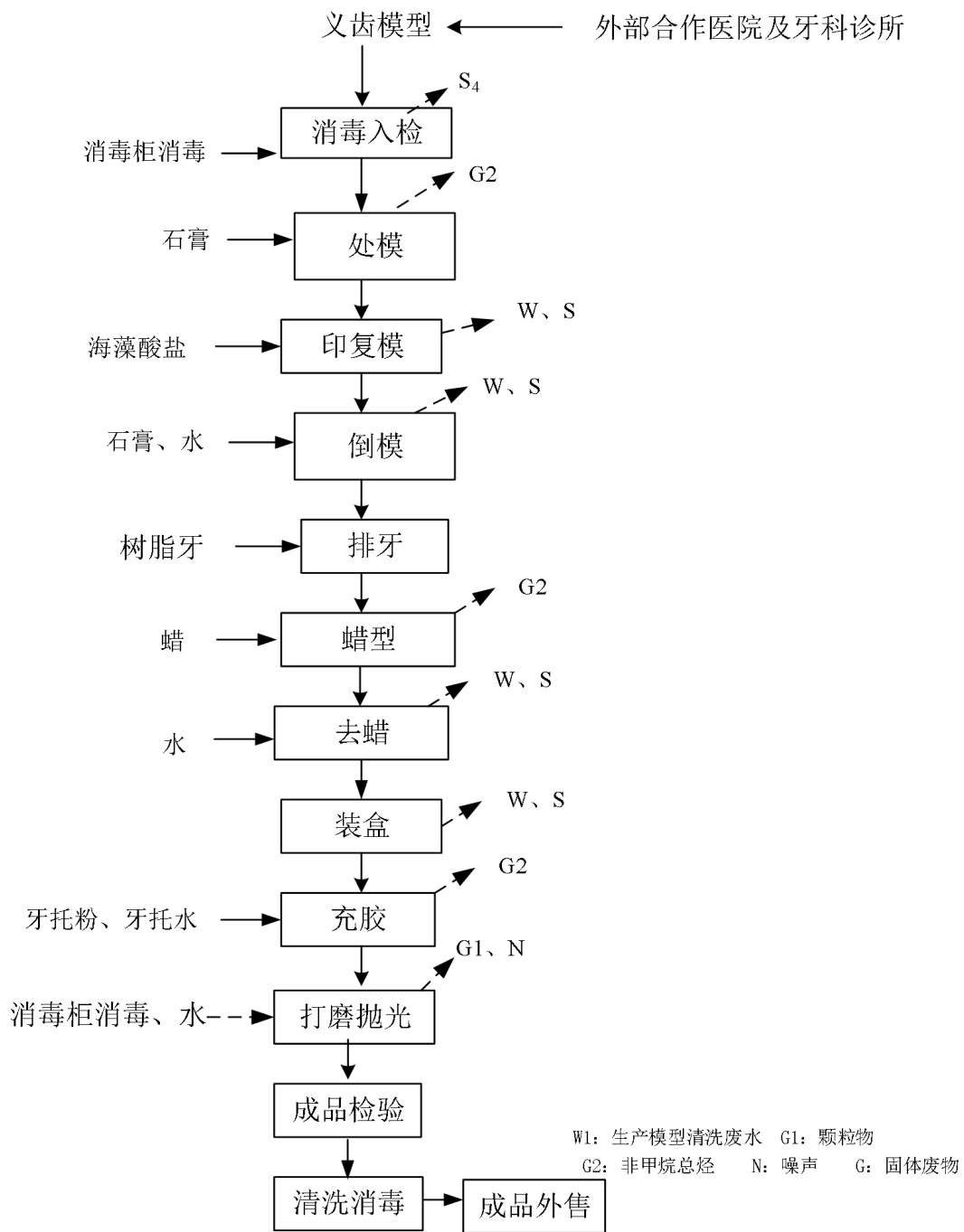
图 2-7 活动类胶托类义齿生产工艺流程及产污节点
