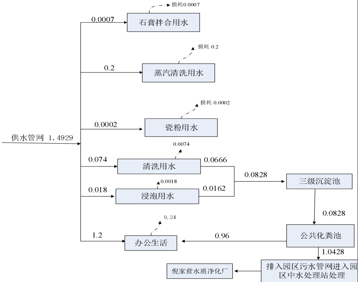
图 2-1 运营期水平衡示意图 单位：m³/d
