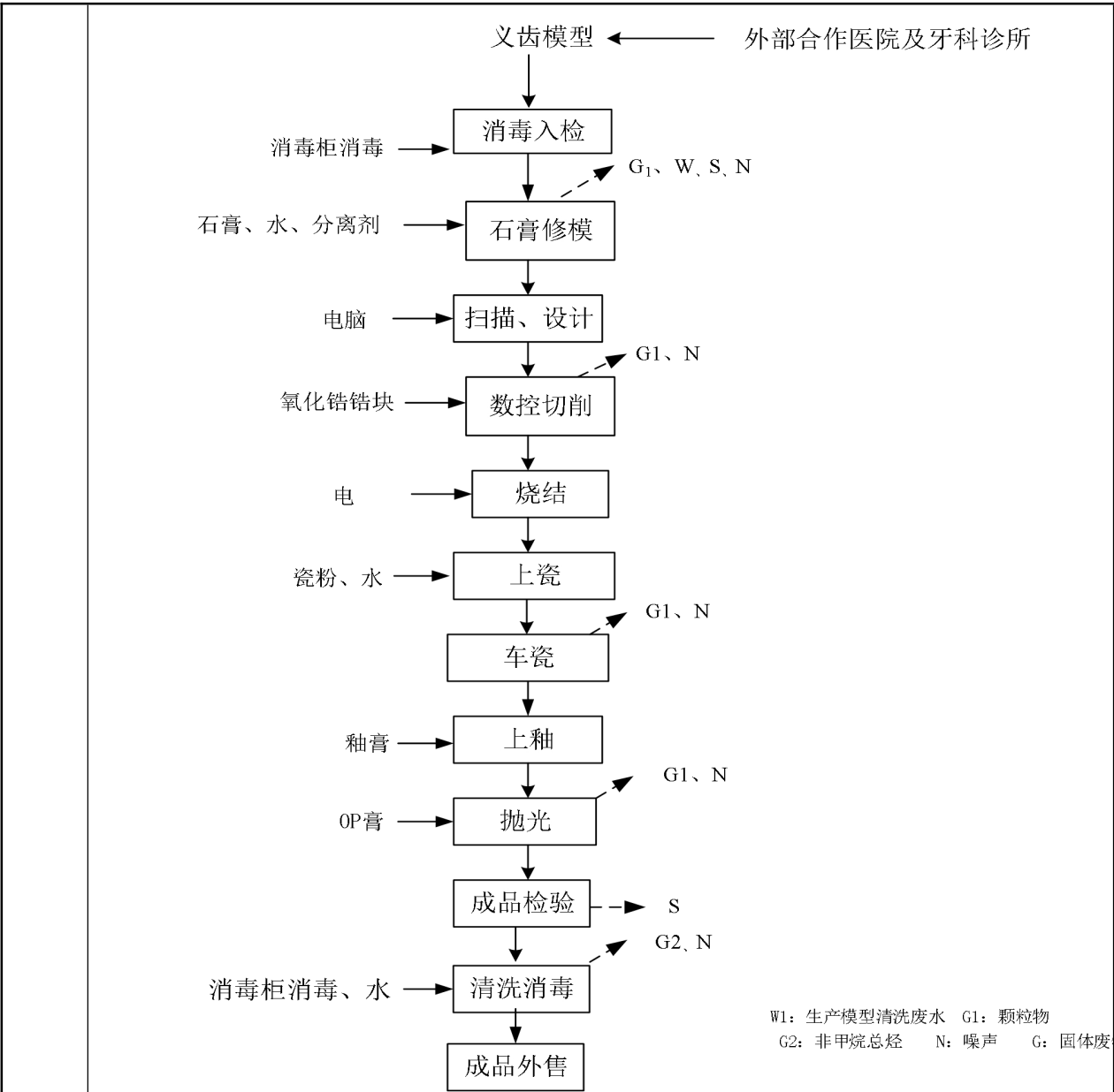
图 2-4 固定类全瓷类义齿生产工艺流程及产污节点示意图
