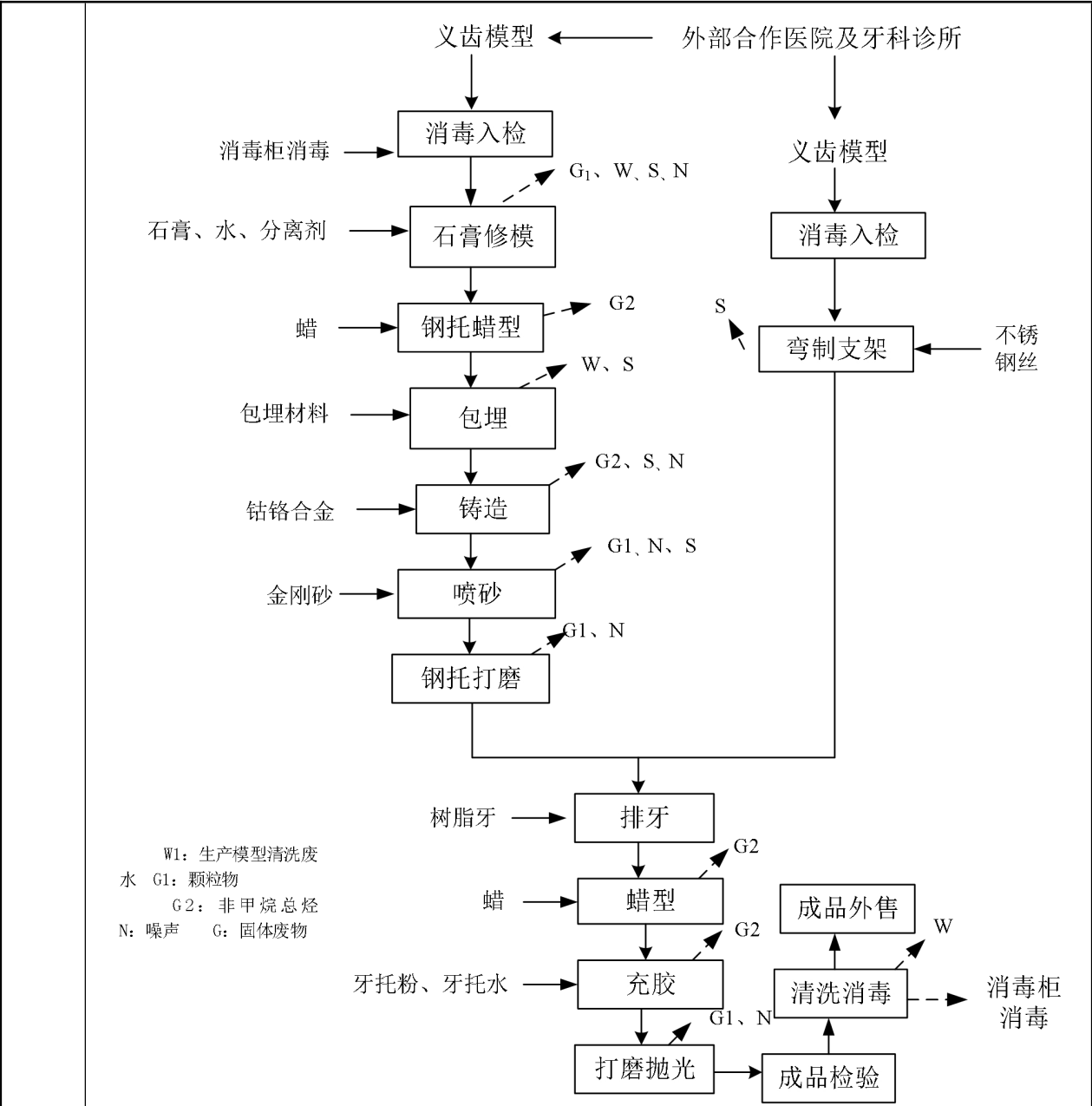
图 2-6 活动类钢托义齿生产工艺流程及产污节点
