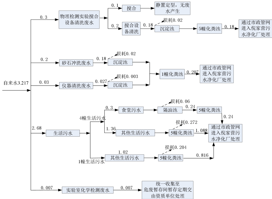
图 2.4-1 项目水量平衡图（单位：m³/d）
