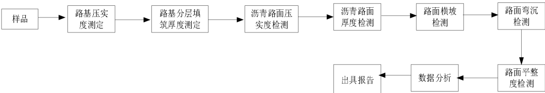
2.9-12 项目路基路面试验工艺流程
