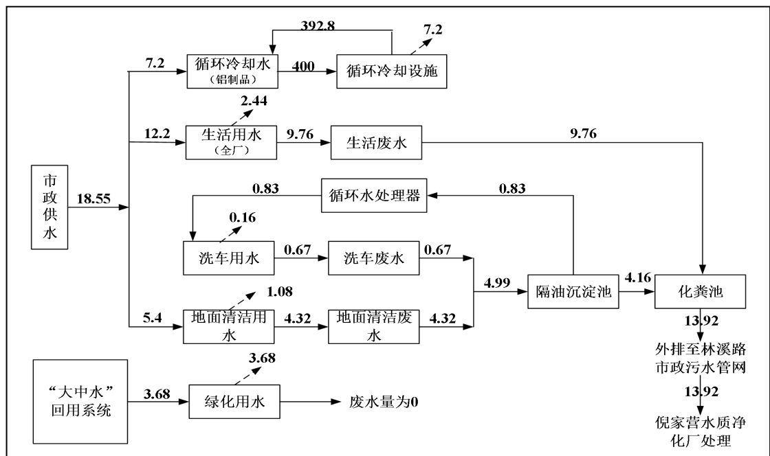
图 2-1 项目运营期水量平衡图 \text{m}^3/\text{d}
