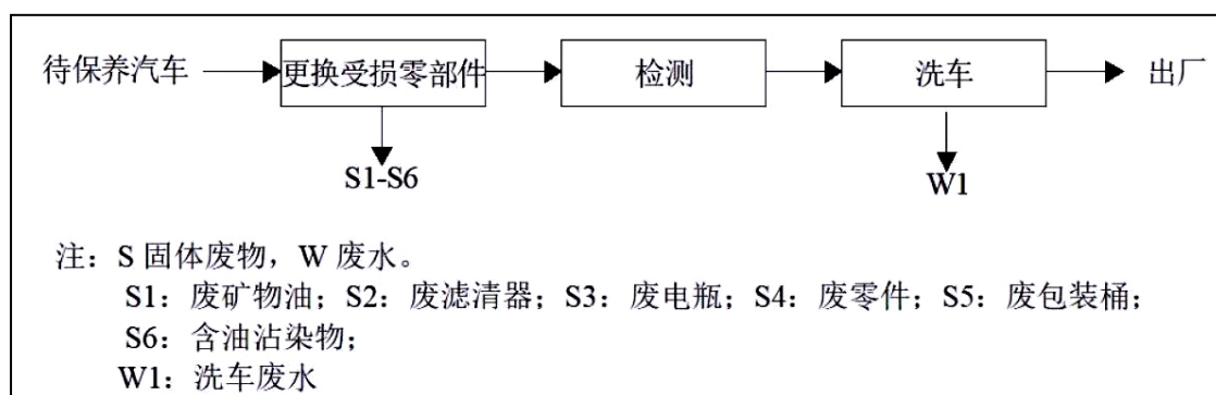
图 2-3 项目内汽车保养工艺流程及产污节点图
