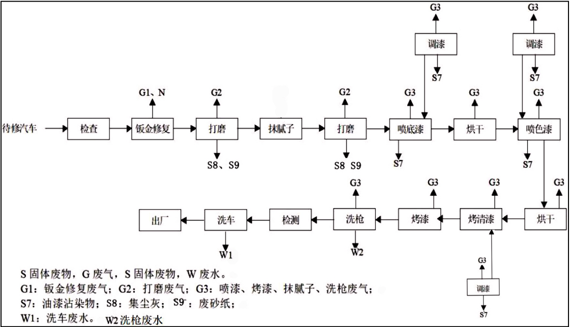
图 2-4 项目内汽车钣喷工艺流程及产污节点图
