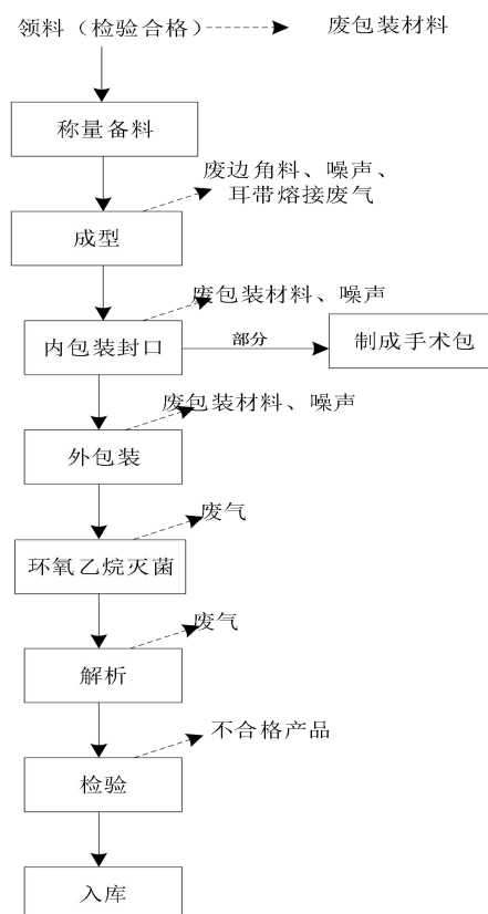
图 2-3 医用防护口罩生产工艺流程及产污节点示意图
