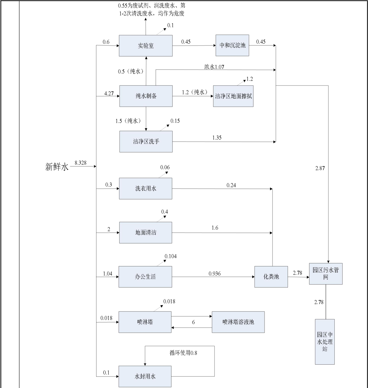
图 2-1 项目水量平衡图 (m³/d)
