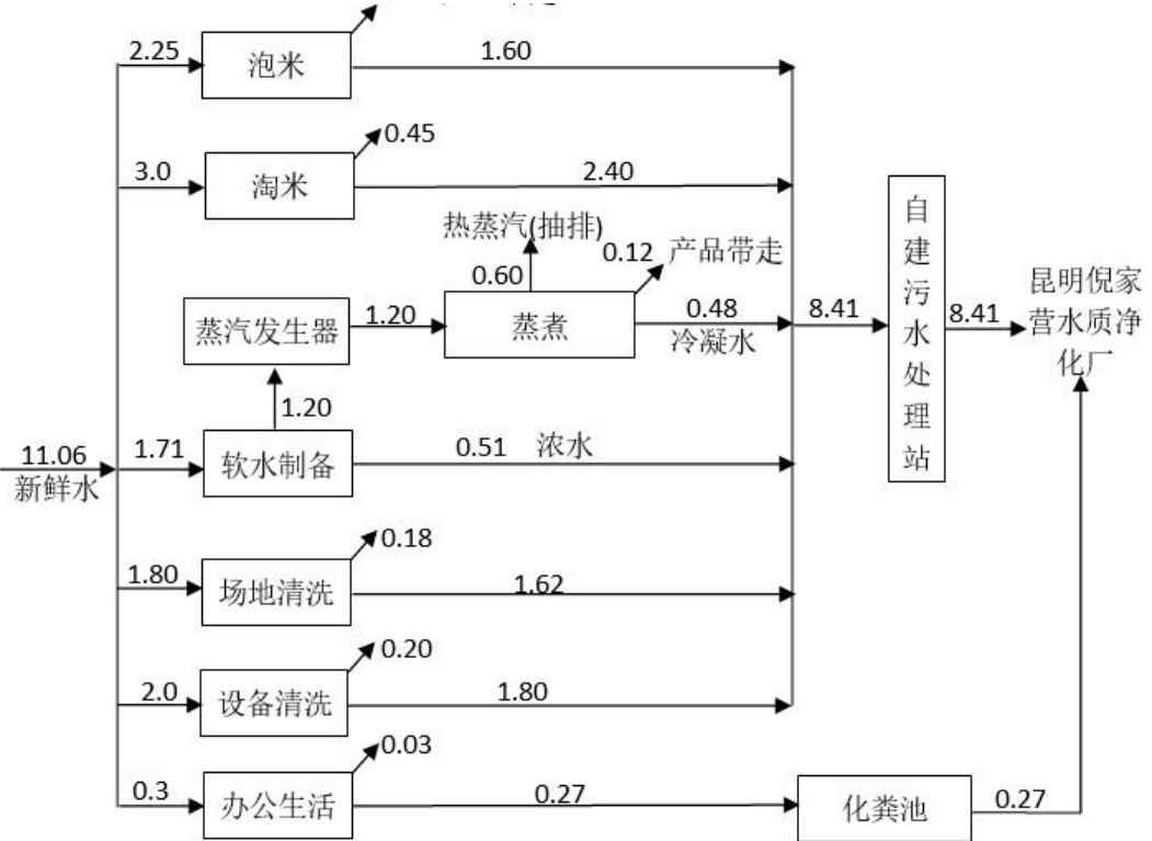
图 2-2 建设项目供排水平衡图(单位: m 3 /d)
