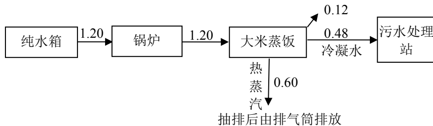
图2-1 建设项目蒸汽平衡一览表(单位: m³/d)
