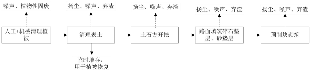
图 4.1-3 至溢洪道控制段道路工程工艺流程及产污节点图
