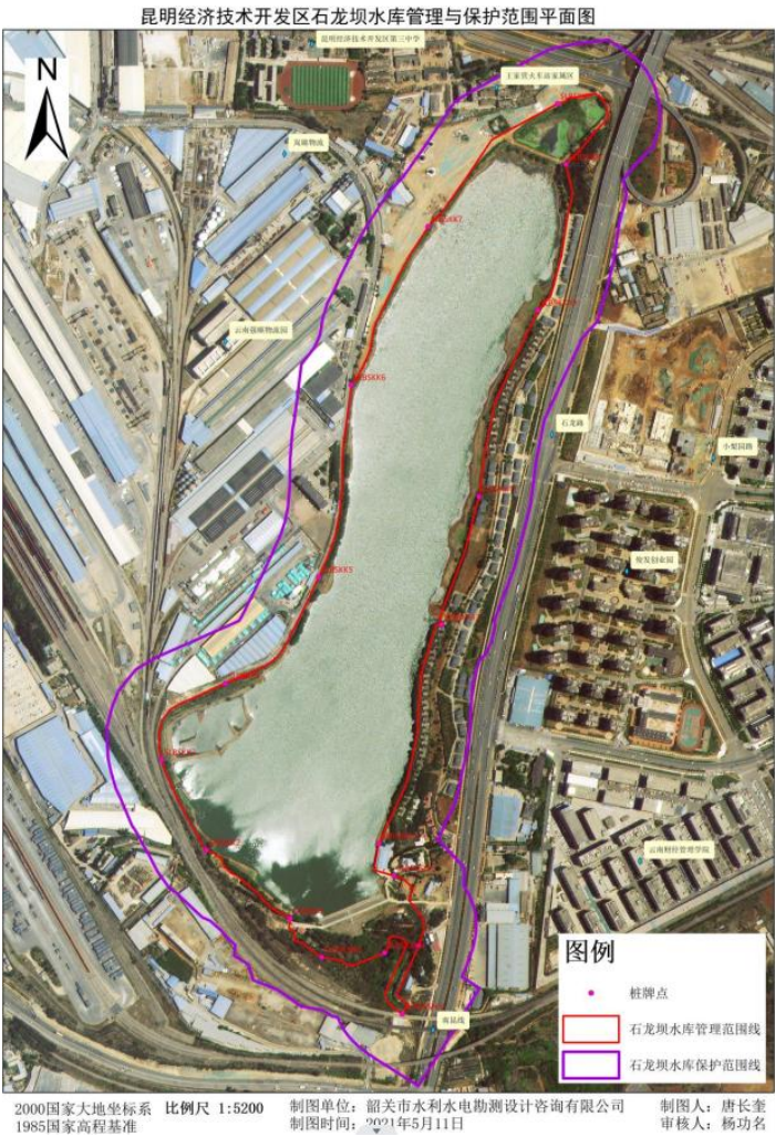
图 2.6-1 石龙坝水库管理范围与保护范围图
