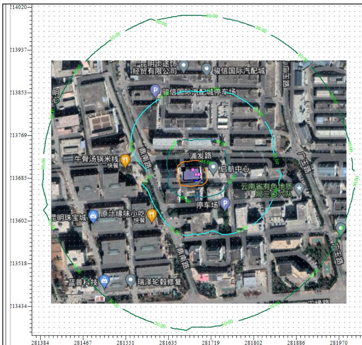
图 4-5 项目运营期噪声等值线图
