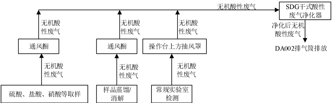
图 4-1 项目运营期无机酸性废气走向示意图
