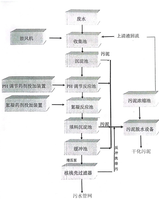
图 4-1 污水处理工艺流程图
