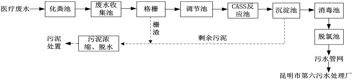
图 4-1 污水处理站工艺流程图
