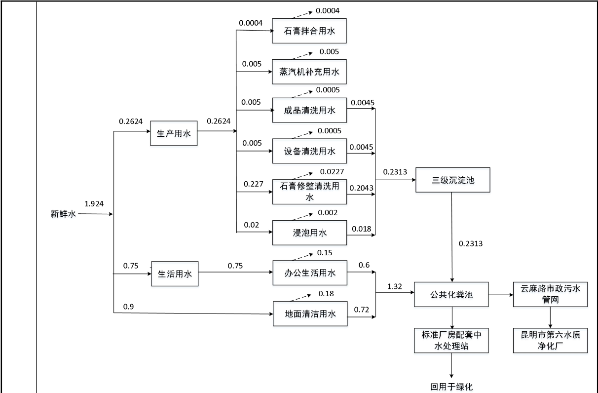
图 2-1 项目水平衡图 \text{m}^3/\text{d}
