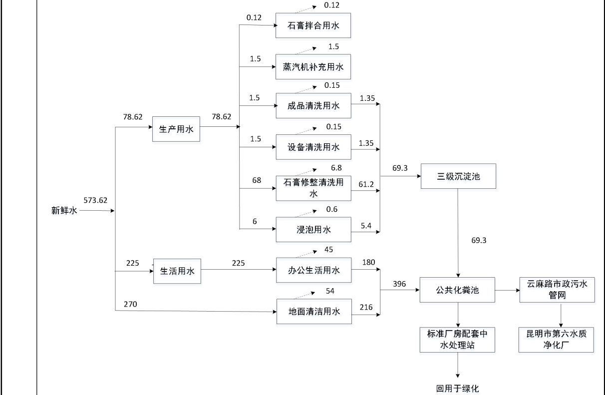
图 2-2 项目水平衡图 \text{m}^3/\text{a}
