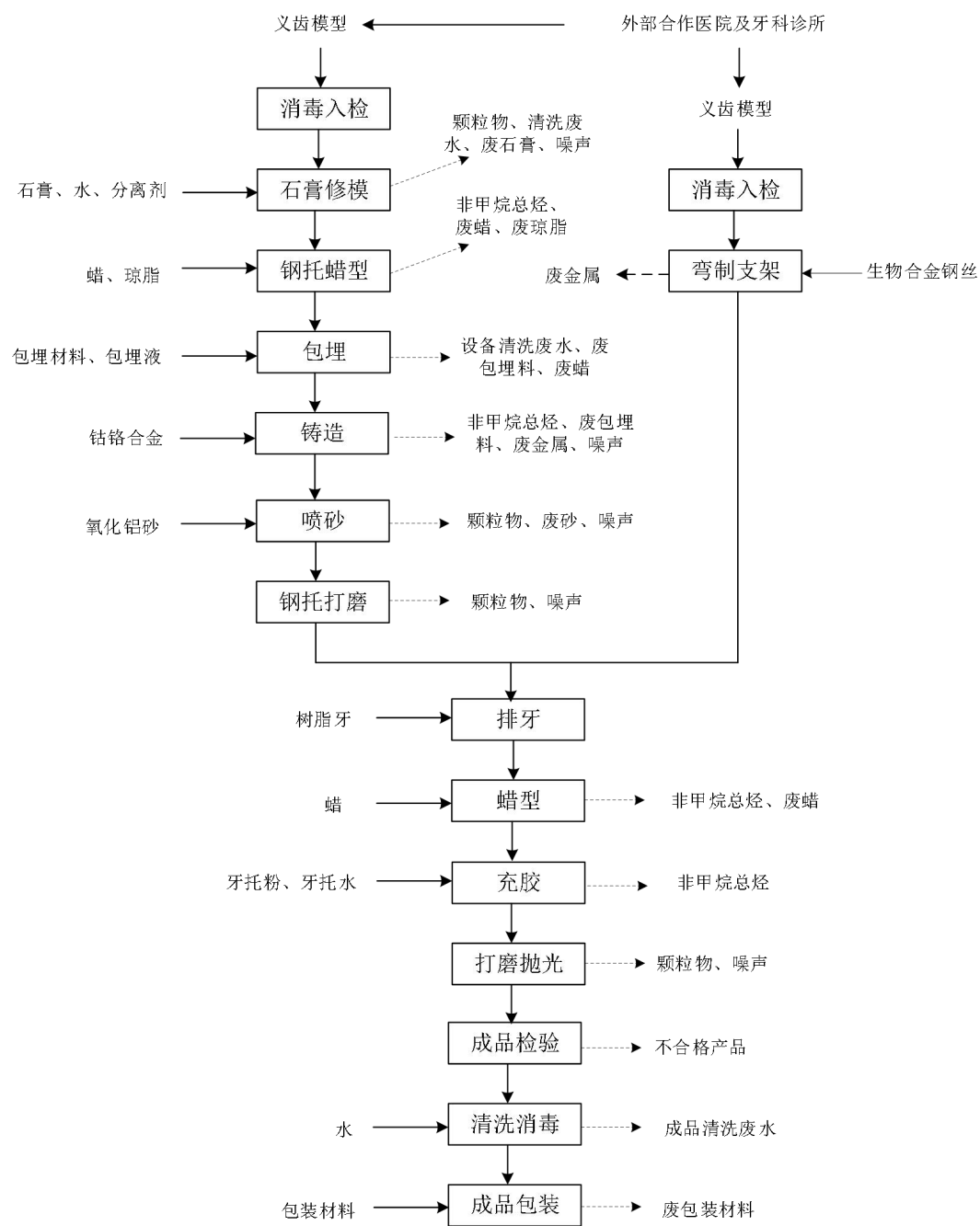
图 2-8 活动类支架类义齿生产工艺流程及产污节点图 工艺流程简述：
