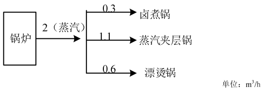
图 2-1 项目蒸汽平衡图（单位 m 3 /h）
