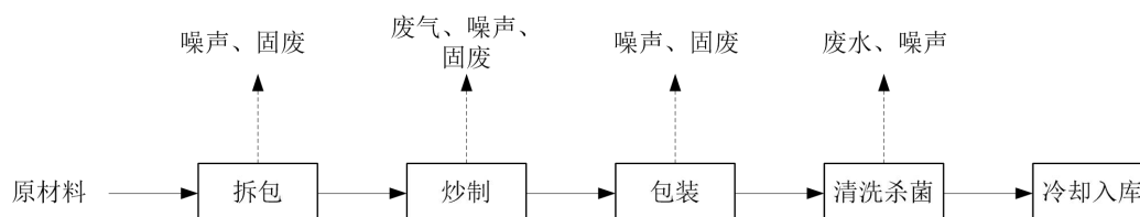
图 2-4 运营期调味品炒制生产工艺流程及产污节点图
