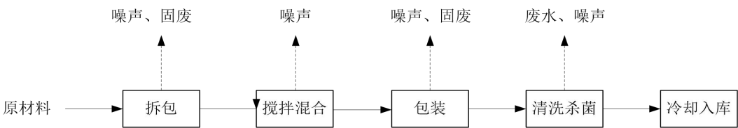
图 2-8 调味品分装生产工艺流程及产污节点图
