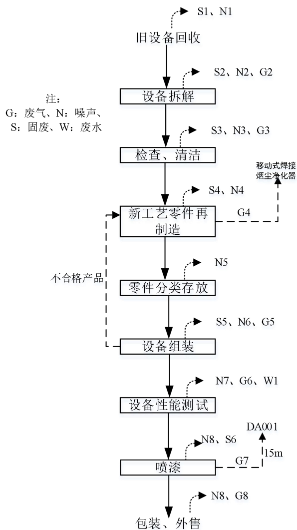
图 2-2 工业泵再制造工艺流程图
