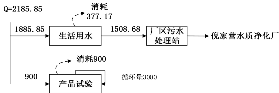
图 2-1 技改扩建后项目水量平衡图 单位：m³/a
