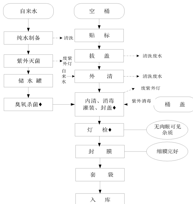
图 2-17 饮用水生产工艺流程图及产污节点图
