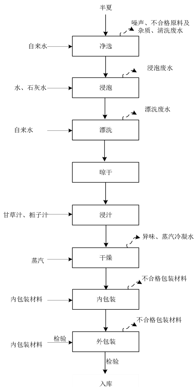
图 2-12 京半夏生产工艺流程及产排污节点图
