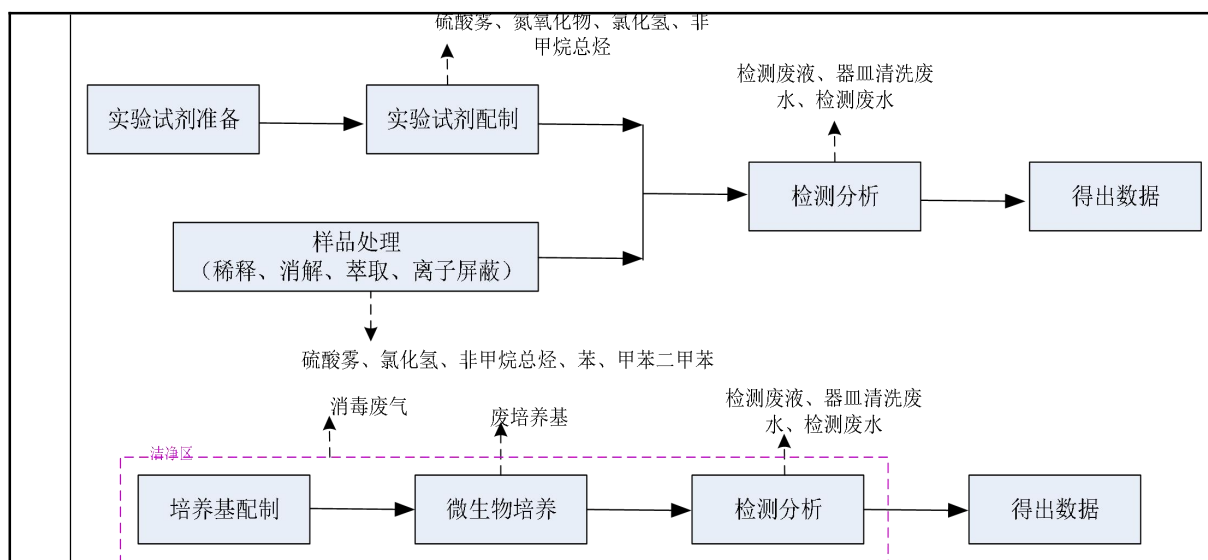
图 2-20 项目质检、检验流程及产污节点图
