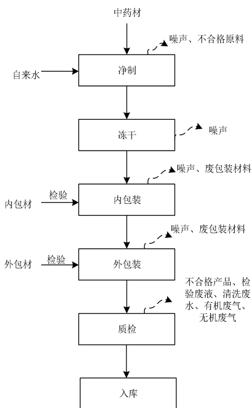
图 2-8 冻干中药饮片生产工艺流程及产污环节图
