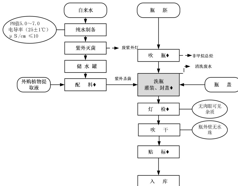
图 2-18 植物饮料生产工艺流程图
