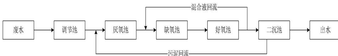
图 4-1 污水处理站处理工艺流程图
