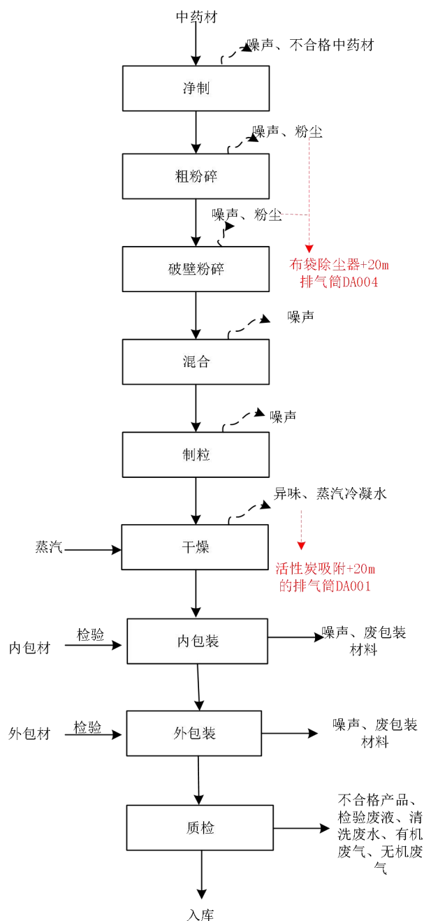
图 2-9 破壁中药饮片生产工艺流程及产污节点图 工艺流程简述：
