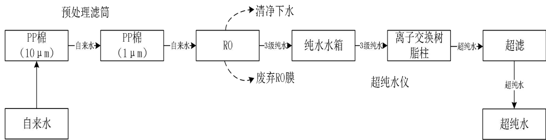
图 2-3 纯水制备工艺流程图
