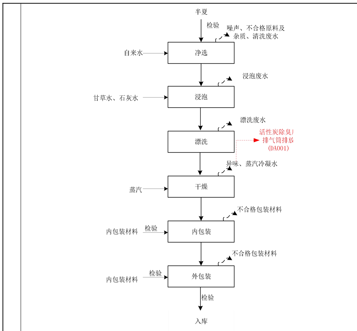
图 2-10 法半夏生产工艺流程及产排污节点图
