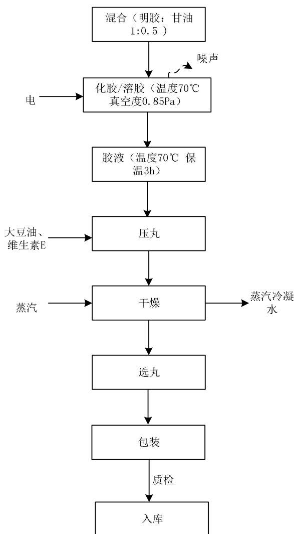
图 2-14 软胶囊保健品生产工艺流程图
