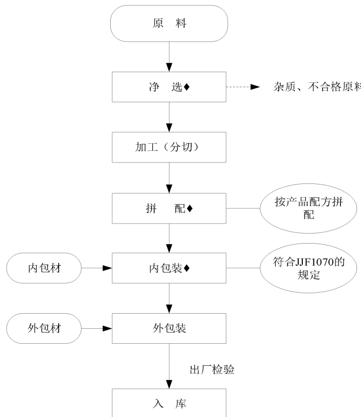
图 2-15 大健康代用茶、汤料、蔬菜制品生产工艺流程及产污节点图
