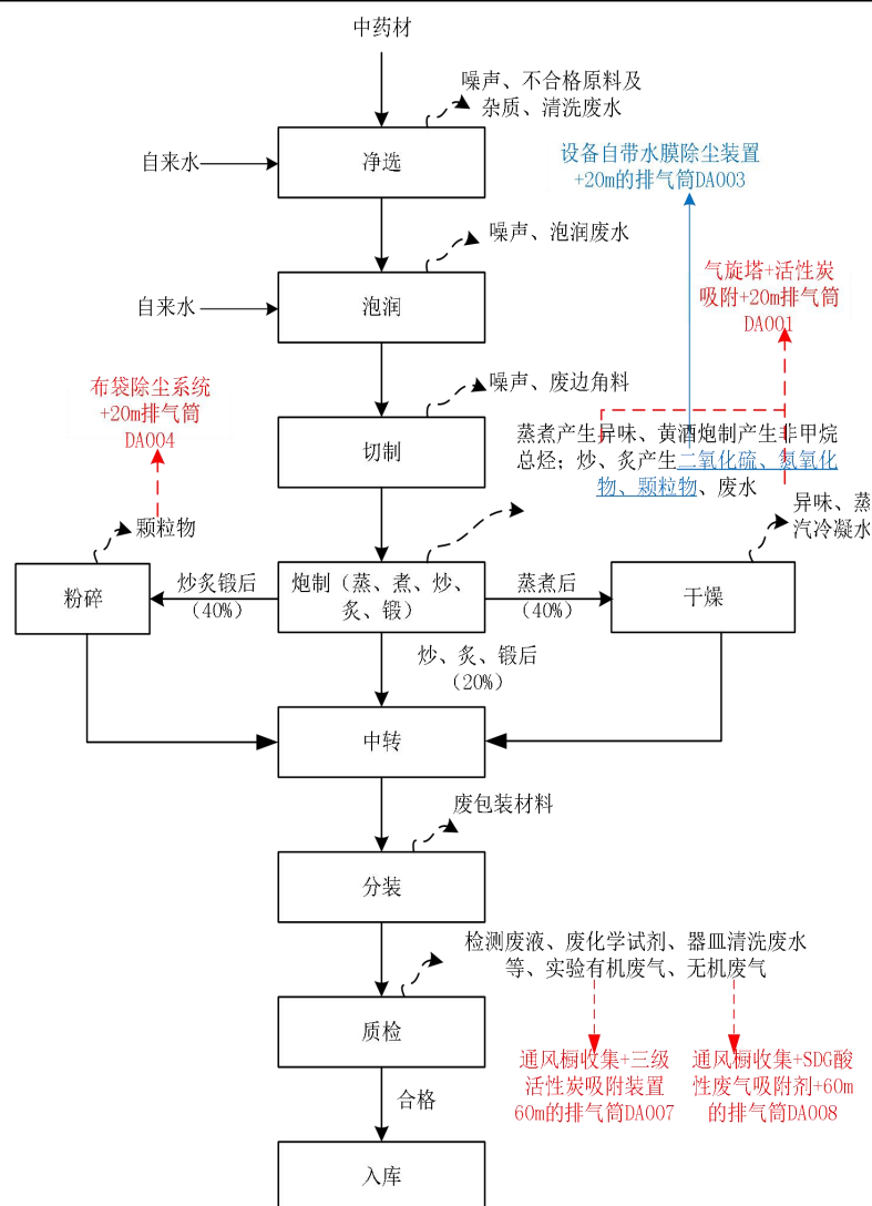
图 2-6 普通、精制、贵细中药饮片生产工艺流程及产污节点图
