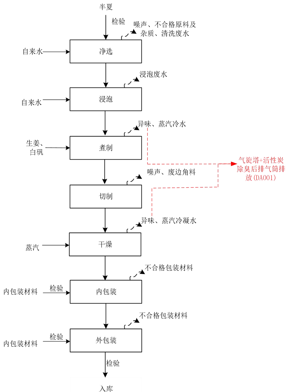
图 2-11 法半夏生产工艺流程及产排污节点图
