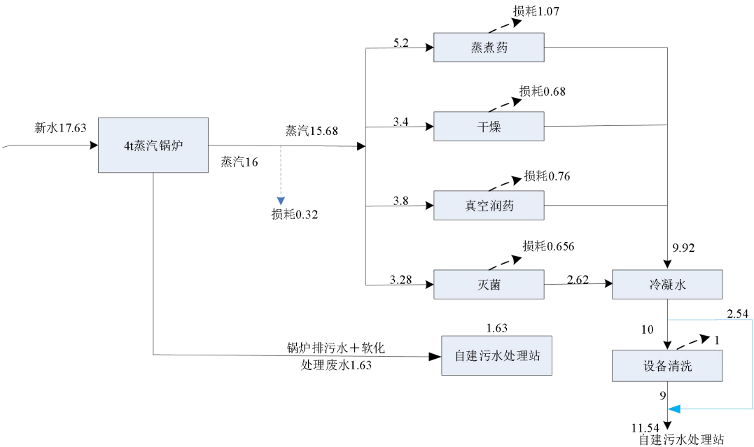
图 2-1 生产线天然气锅炉蒸汽平衡图 (t/d)
