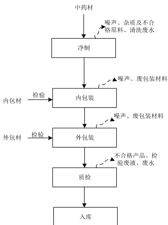
图 2-13 三七天麻等生产工艺流程及产排污节点图
