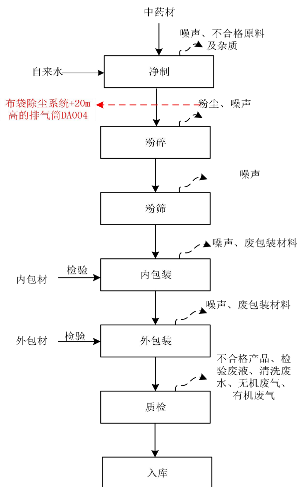
图 2-7 直接口服中药饮片（粉剂）生产工艺流程及产污节点图
