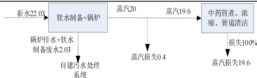
图 2-2 智慧中药房天然气锅炉蒸汽平衡图 (t/d)
