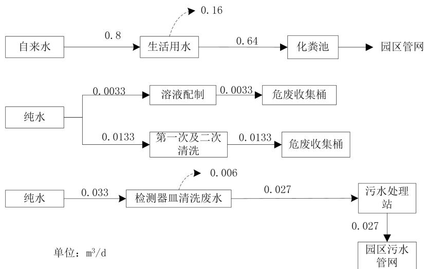
图 2-1 项目日水量平衡图
