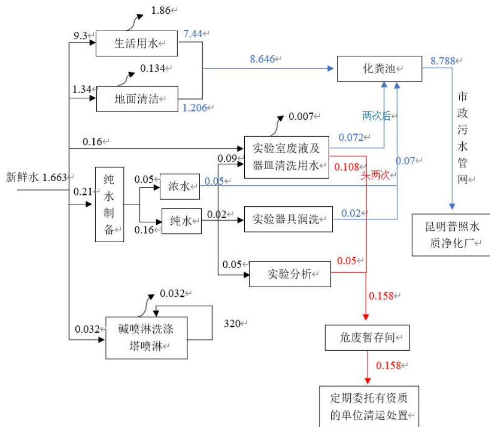
图 2-1 项目平衡图 单位 m³/d
