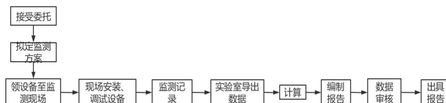
图 2-7 运营期现场监测项目工艺流程图
