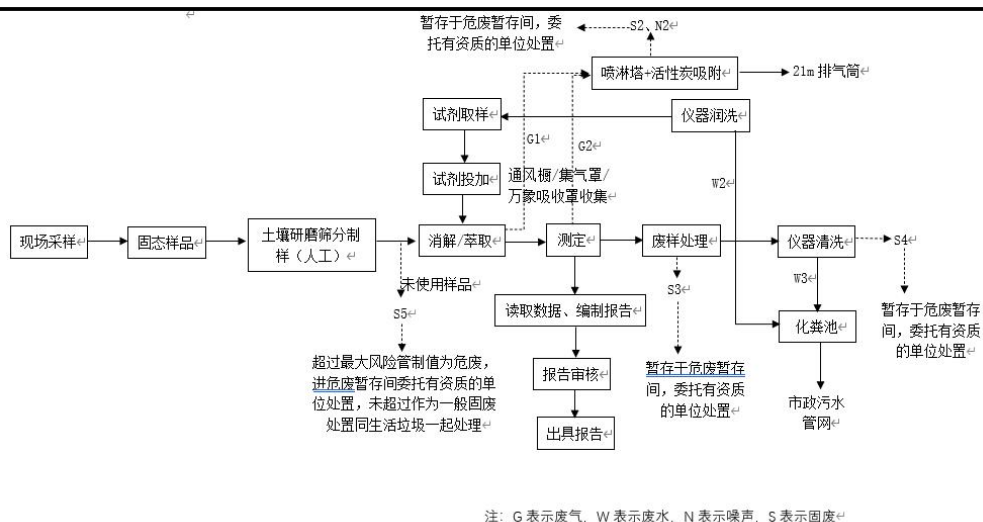
图 2-5 运营期固态样品检测流程及产污节点工艺流程图
