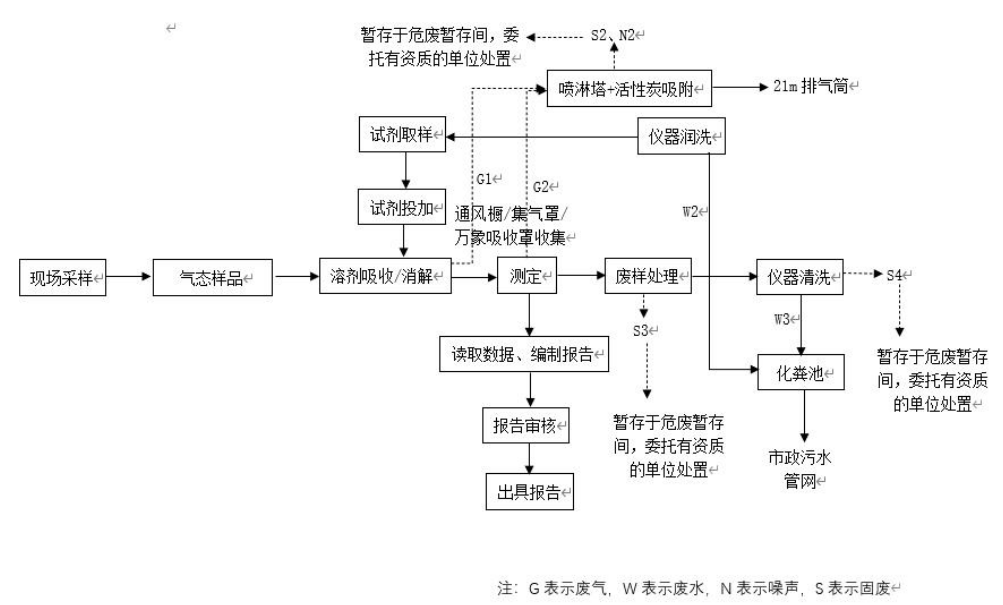
图 2-4 运营期气态样品检测流程及产污节点工艺流程图
