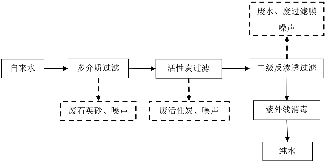
图 2-7 项目纯水制备流程及污染工序图
