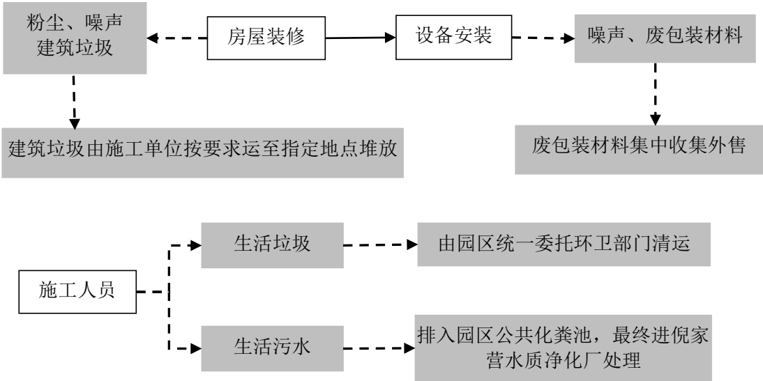
图 2-2 施工工艺流程及污染工序图
