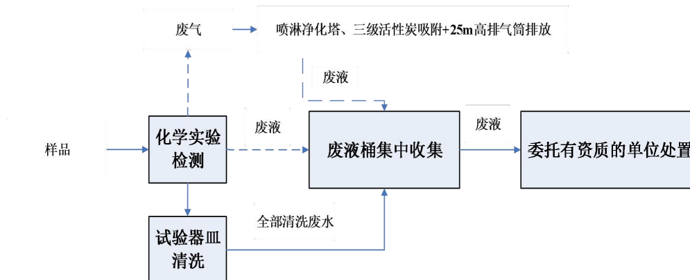
图 2-2.1 运营期化学实验工艺流程及产污环节示意图
