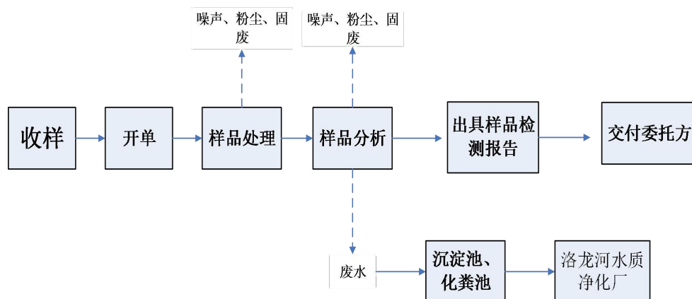
图 2-1 运营期物理实验工艺流程及产污环节示意图
