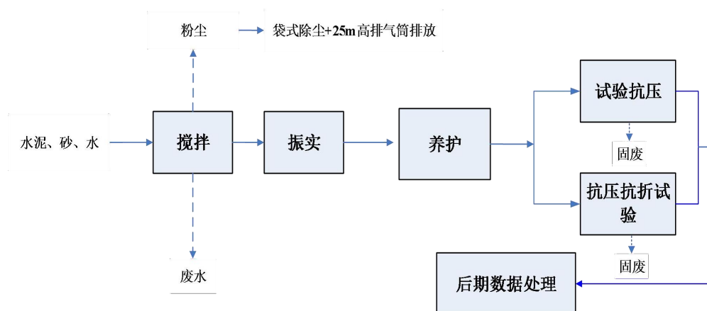
图 2-1.2 水泥混凝土试验流程图
