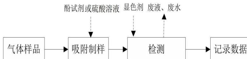
图 2-2.2 空气中甲醛、氨测定工艺流程
