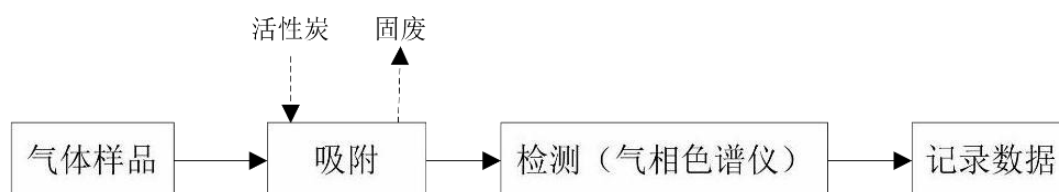
图 2-2.3 空气中苯、甲苯、二甲苯和 TVOC 测定工艺流程
