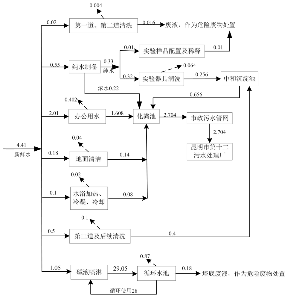
图 2-2 项目水量平衡图（单位：m³/d）
