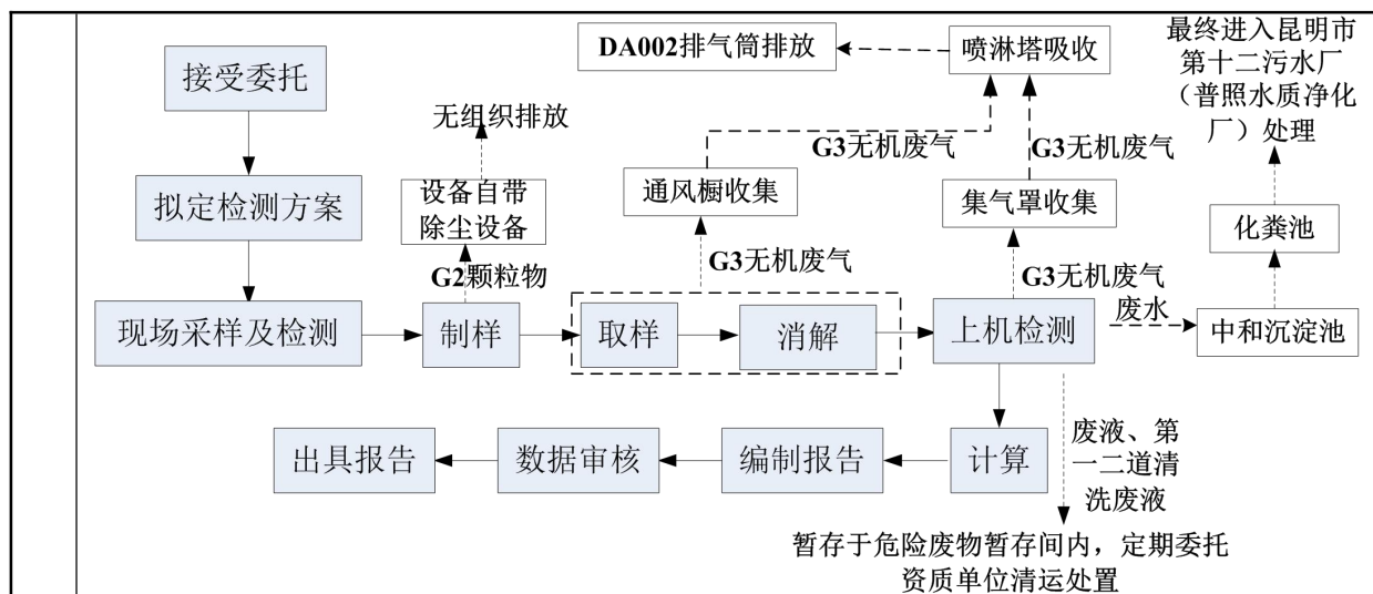
图 2-5 项目运营期无机实验工艺流程及产污环节示意图
