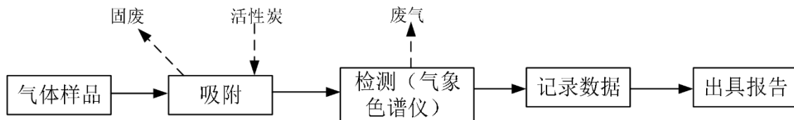
图2-11 空气中苯、甲苯、二甲苯和 TVOC 测定工艺流程及产污环节图
