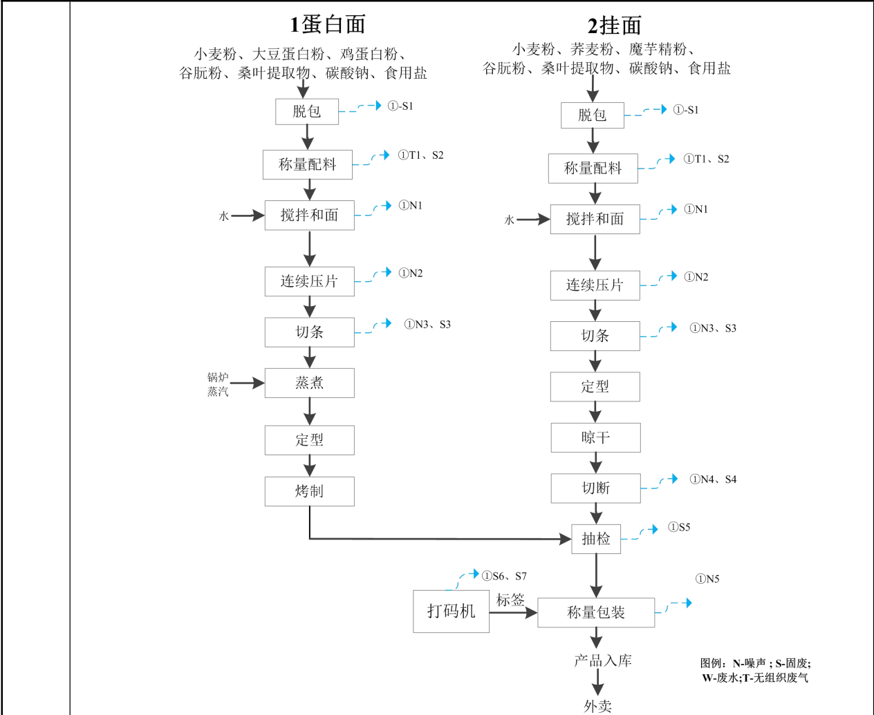
图 2-3 面条生产线工艺流程及产污环节图
