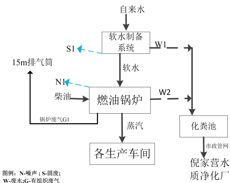
图 2-7 锅炉生产工艺流程图
