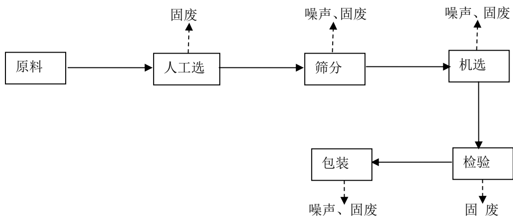
图 2-10 青葱、山葵叶工艺流程及污染工序图
