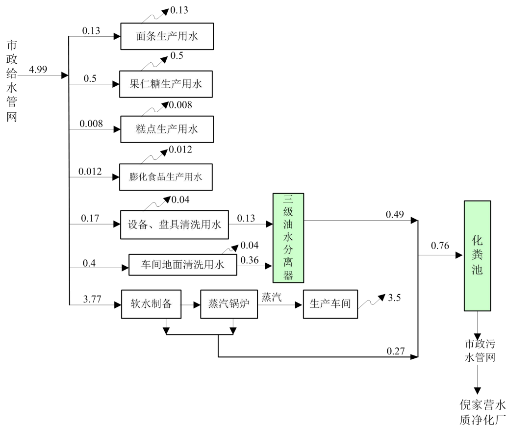
图 2-1 项目水量平衡图 (单位: \text{m}^3/\text{d} )
