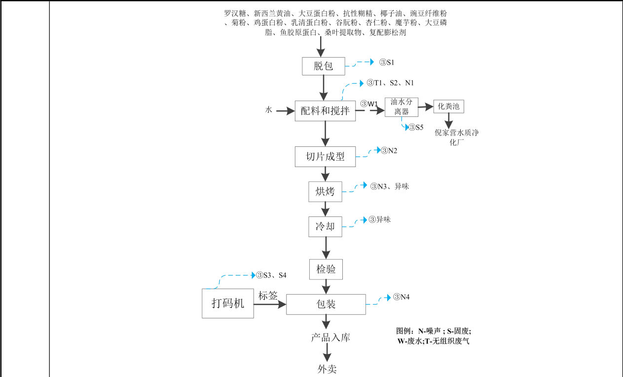
图 2-5 糕点生产线工艺流程及产污环节图
