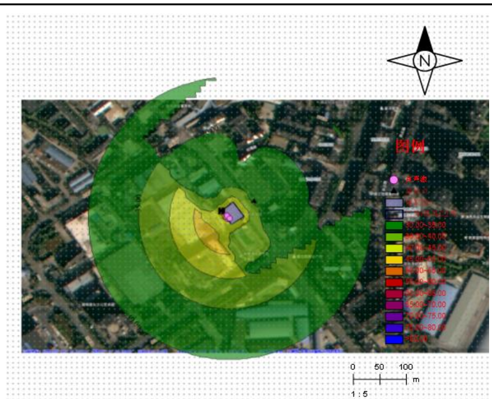
图 4-1 项目等声值线图
