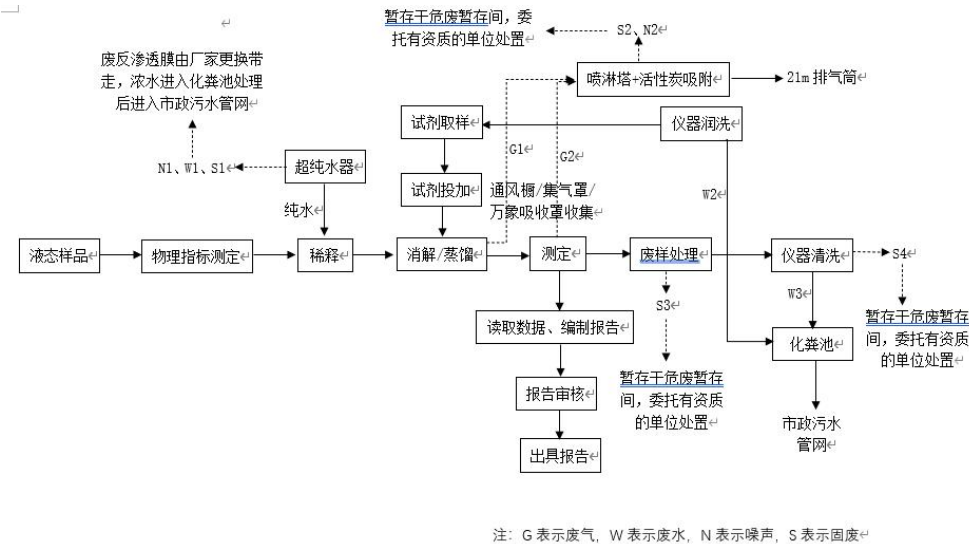
图 2-3 运营期液态样品检测流程及产污节点工艺流程图
