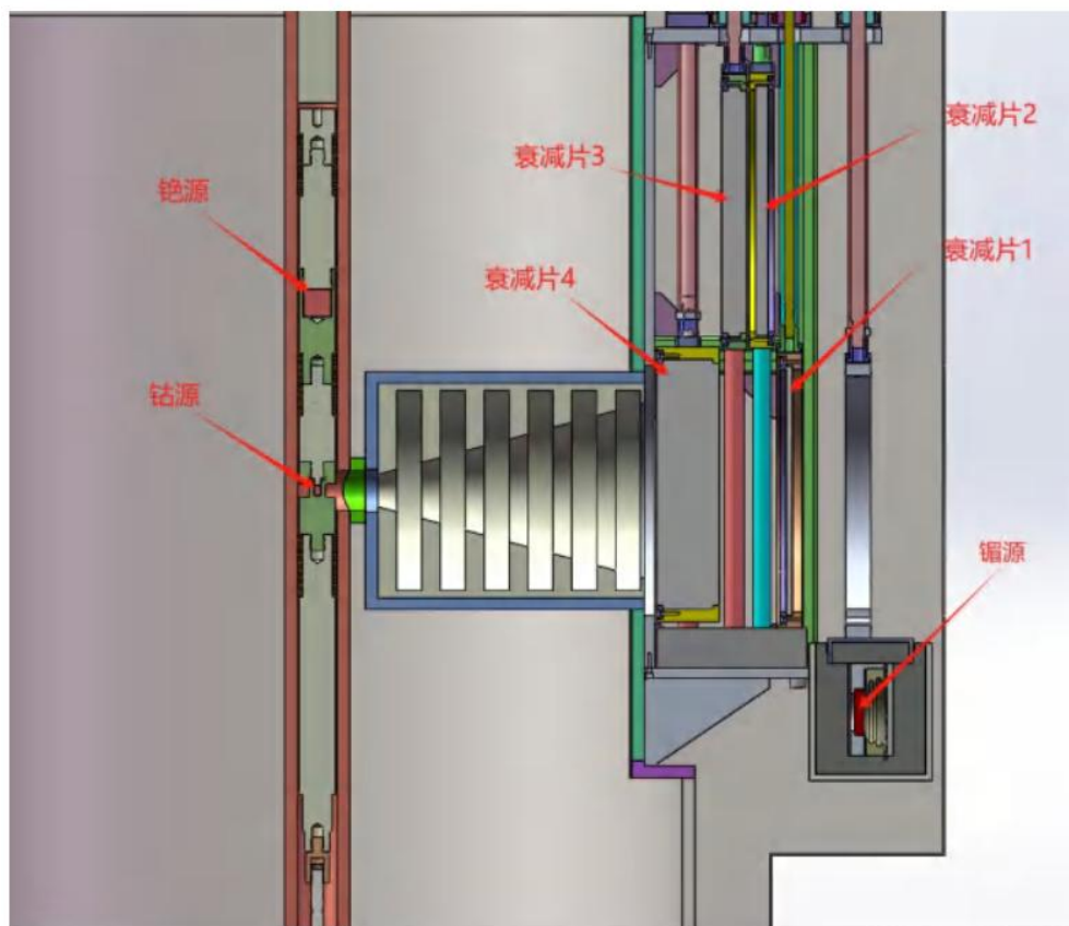
图 2-10 \gamma 射线检定装置内部结构图
