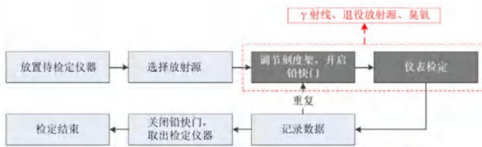
图 2-12 \gamma 射线系统检定工艺流程及产污位置图
