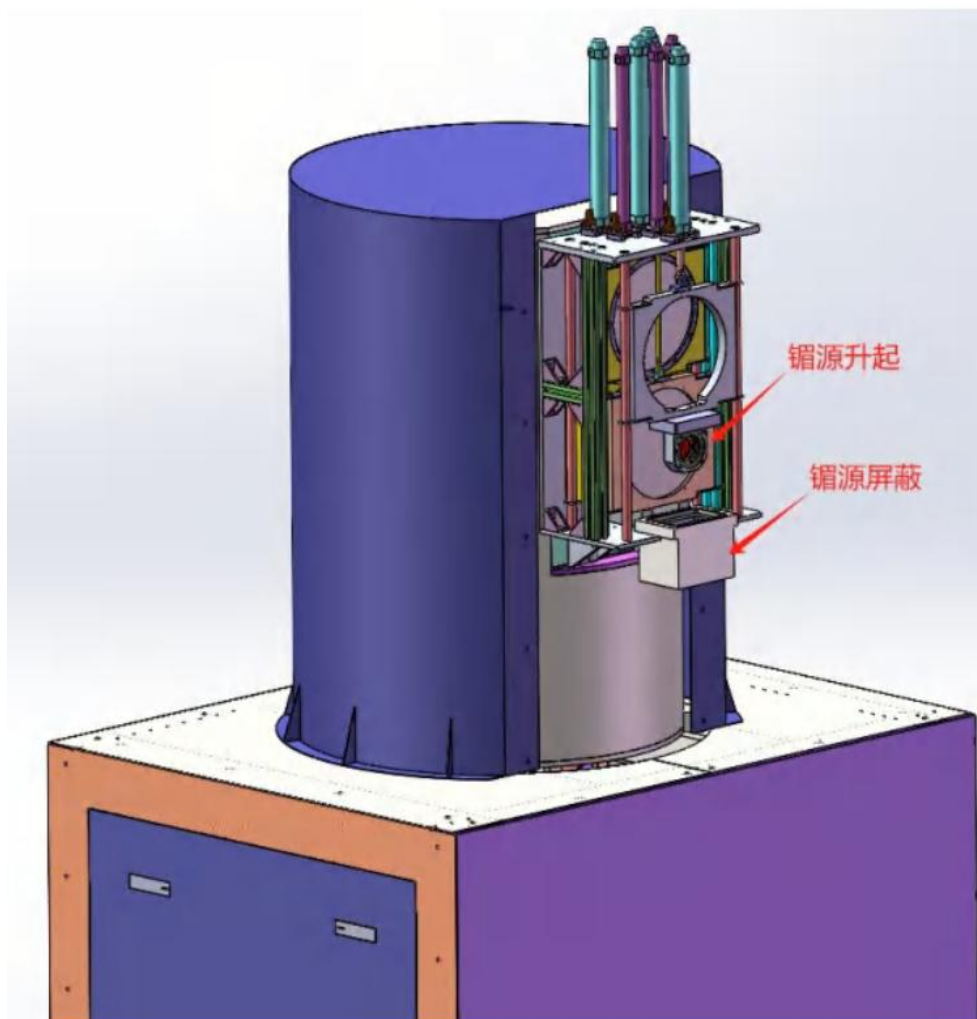
图 2-11 \gamma 射线检定装置设备外形示意图
