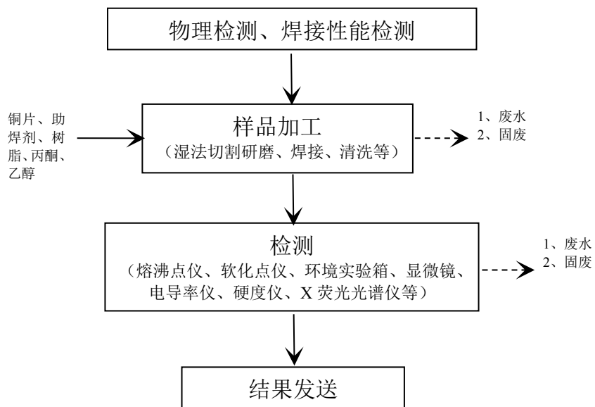
图 2-9 分析实验工艺流程及产污节点图
