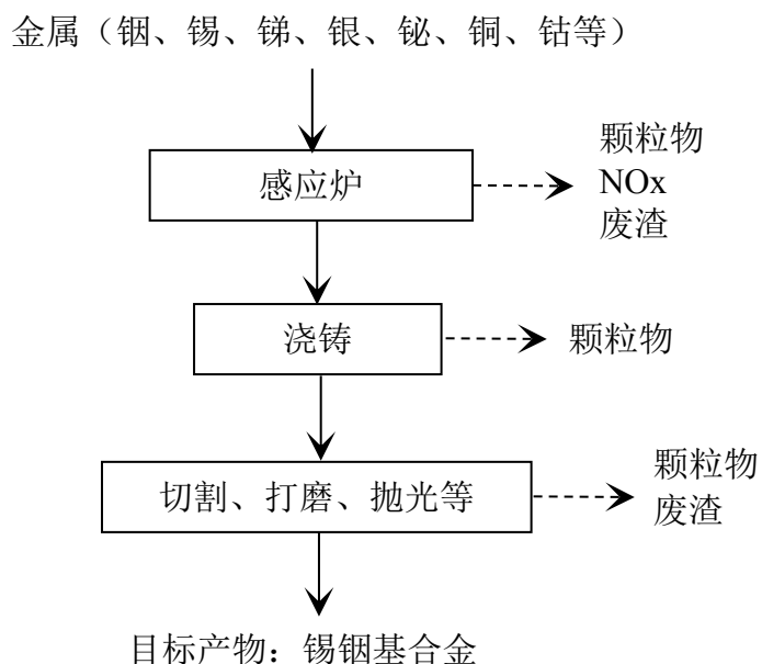
图 2-2 锡铟基合金研究工艺流程及产污节点图
