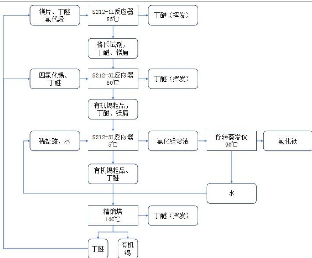
图 2-5 有机锡研究工艺流程及产污节点图
