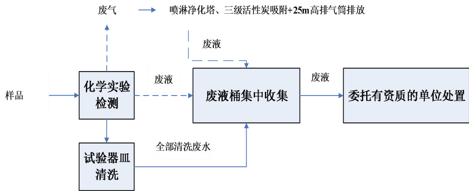
图 2-8 运营期化学实验工艺流程及产污环节示意图
