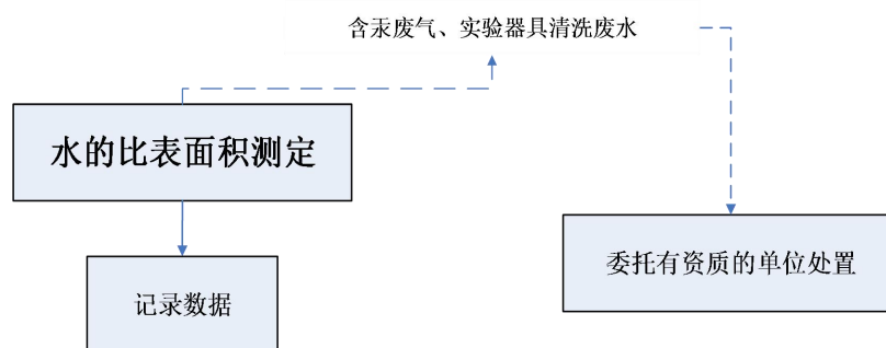
图 2-6 水泥的比表面积测定产污节点图
