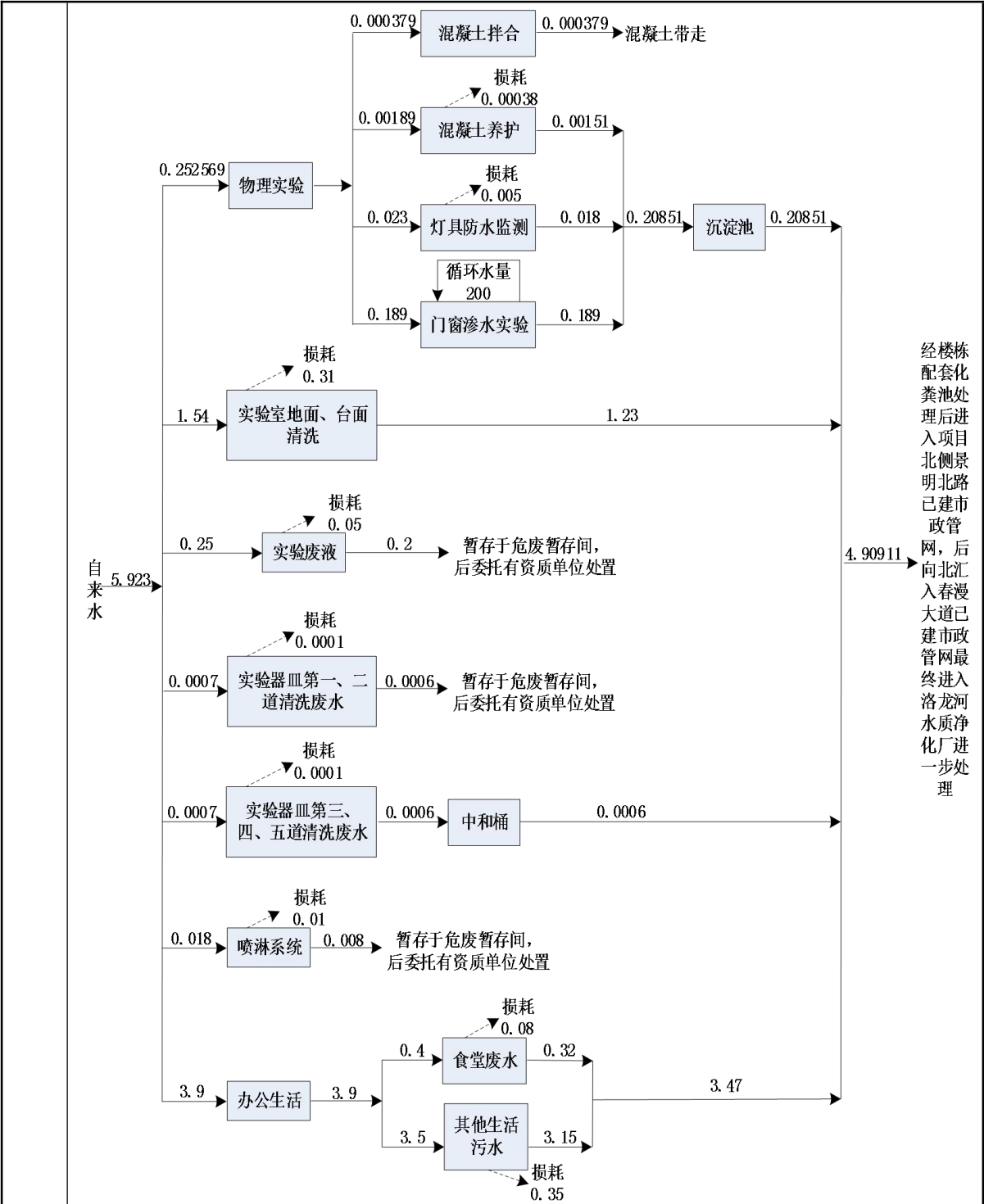
图 4-1 项目水平衡图 单位: m³/d
