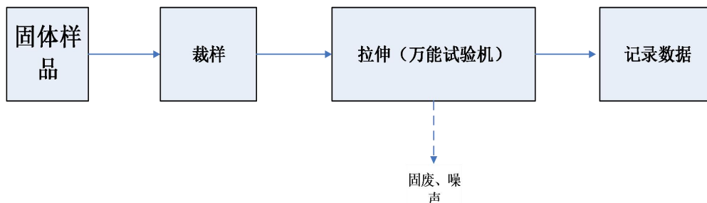
图 2-5 防水材料试验产污节点图
