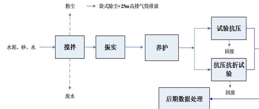
图 2-3 水泥混凝土试验流程图
