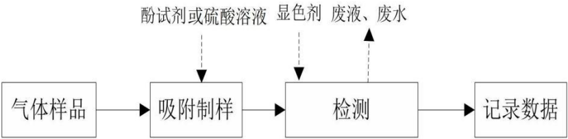
图 2-9 空气中甲醛、氨测定工艺流程
