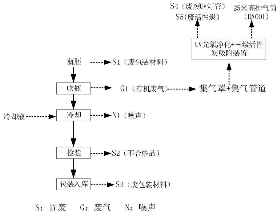
图 2-3 项目 PET 瓶、PET 罐子生产工艺流程及产污节点图
