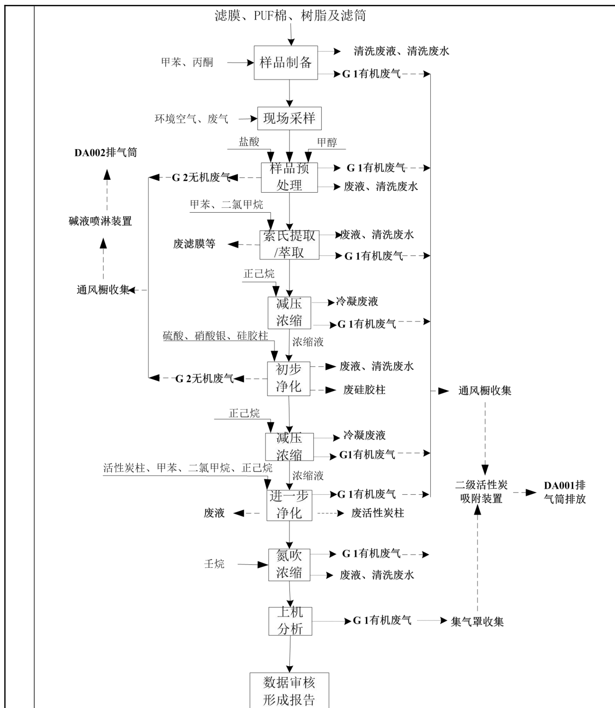
图 2-4 气体样品二噁英检测流程及产污环节示意图
