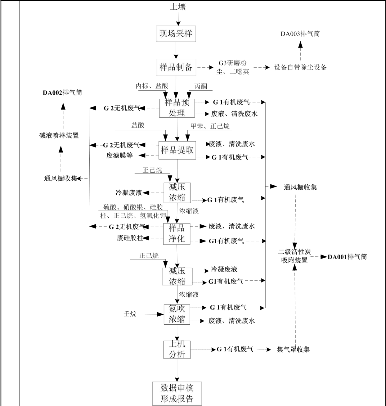
图 2-6 土壤样品二噁英检测流程及产污环节示意图
