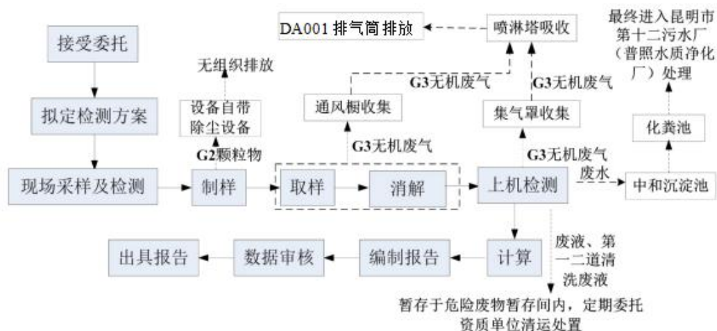
图 2-4 项目运营期无机实验检测流程及产污环节示意图 工艺流程简述：
