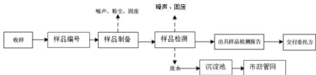
图 2-3 运营期物理实验工艺流程及产污环节示意图
