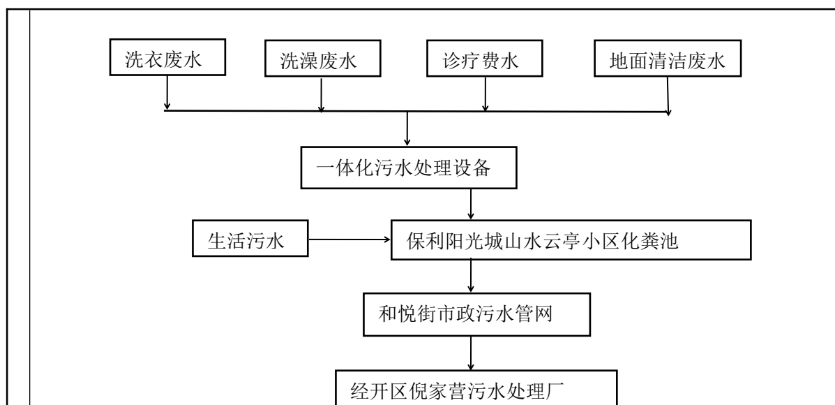
图 4-2 医院污水收集、处理流程
