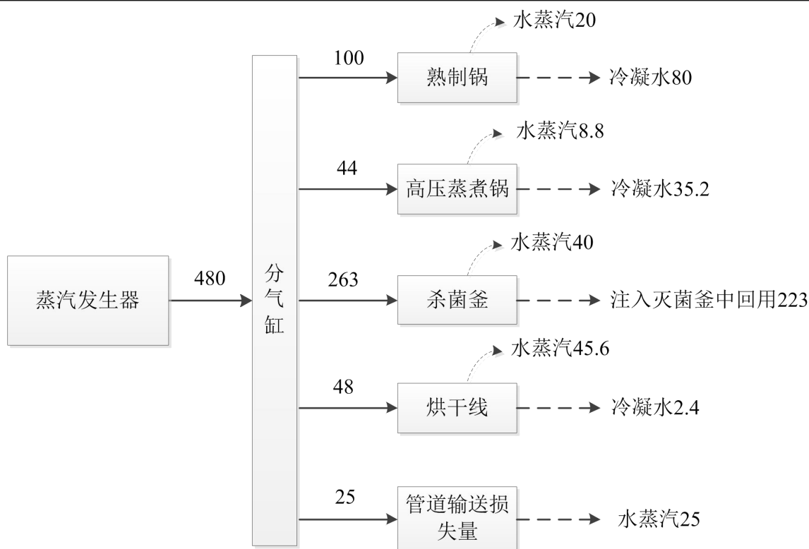
图 2-1 厂区蒸汽平衡图 (t/a)
