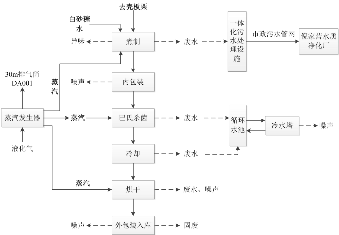
图 2-5 项目煮板栗生产工艺流程及产污节点图
