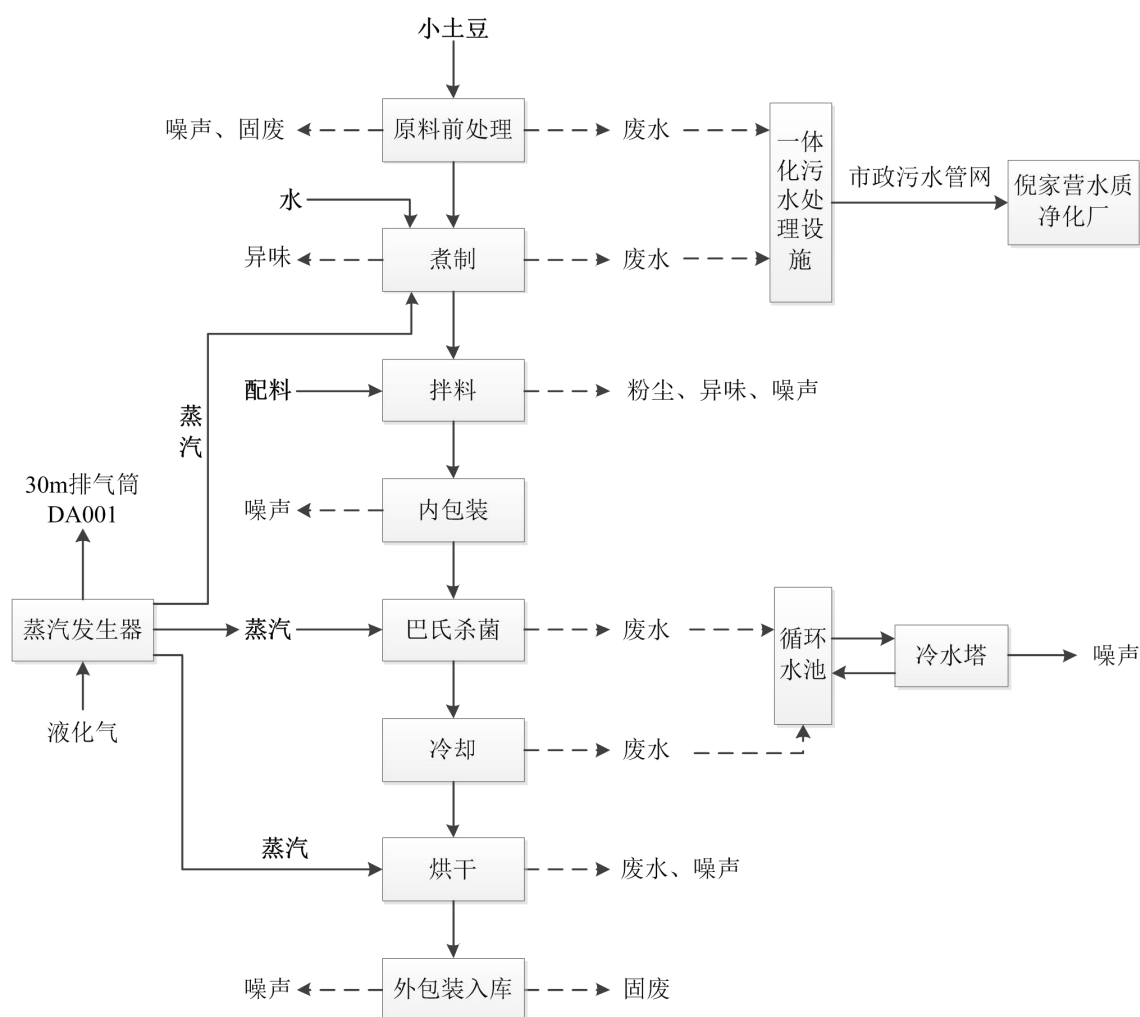
图 2-4 项目高原小土豆生产工艺流程及产污节点图
