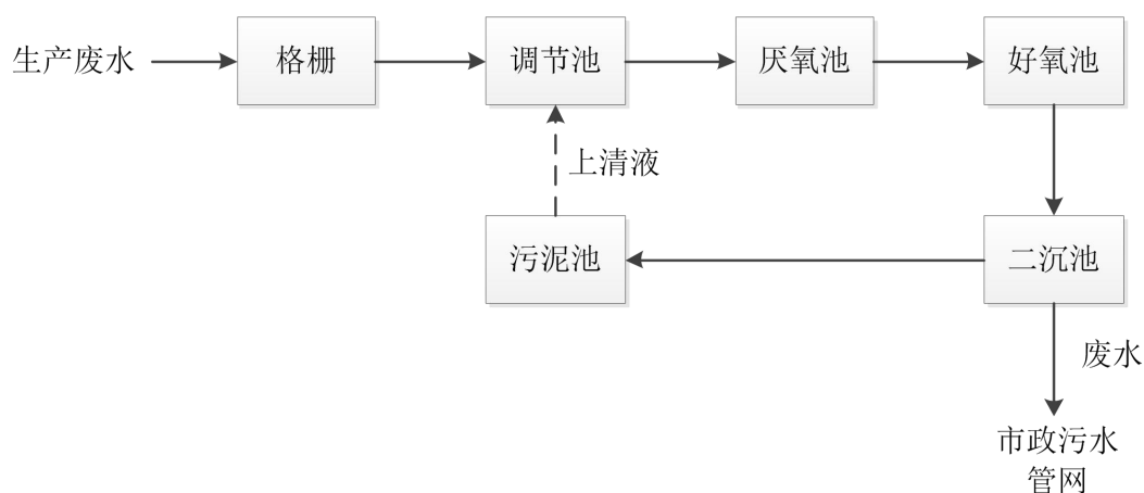
图 4-2 生产废水处理设施流程图
