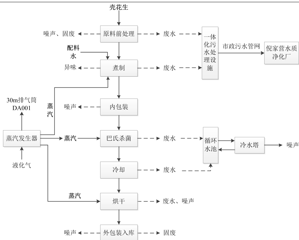
图 2-6 项目卤煮花生生产工艺流程及产污节点图
