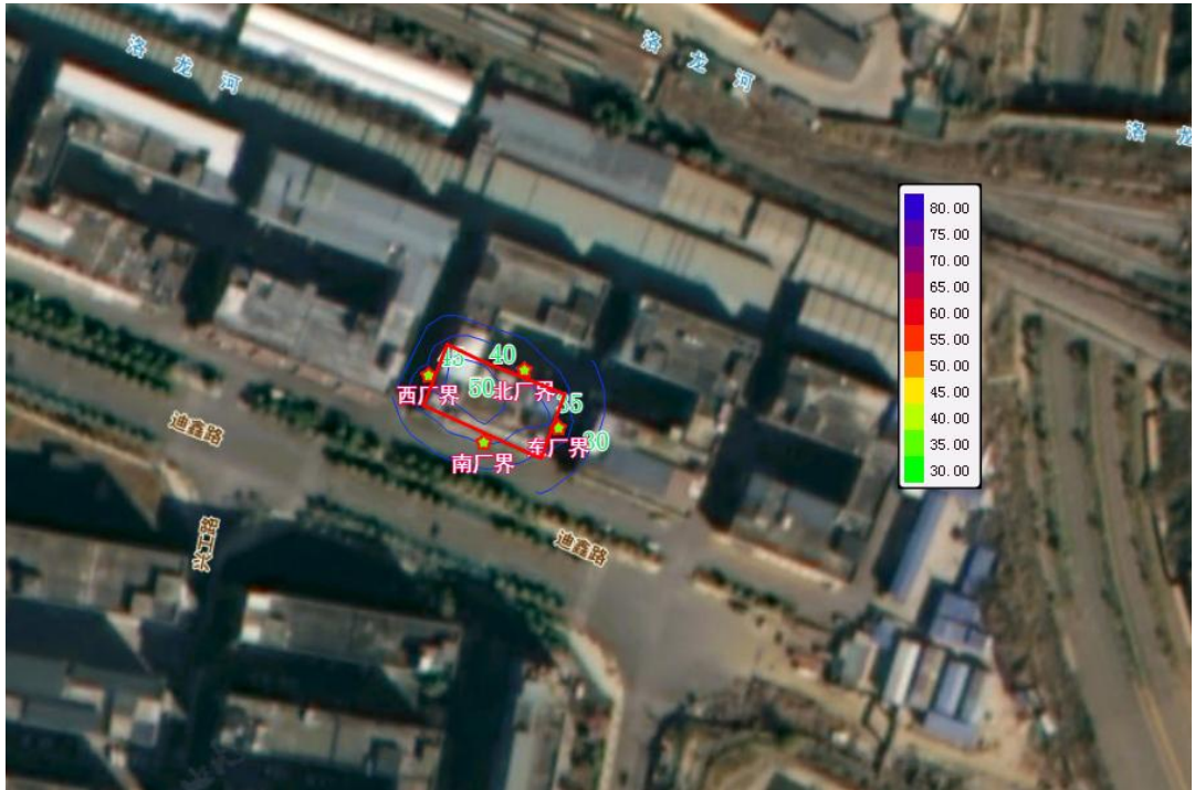
图 4-3 项目噪声贡献等声值线图（昼间）
