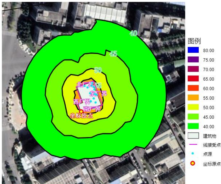
图 4-1 厂界贡献值预测图
