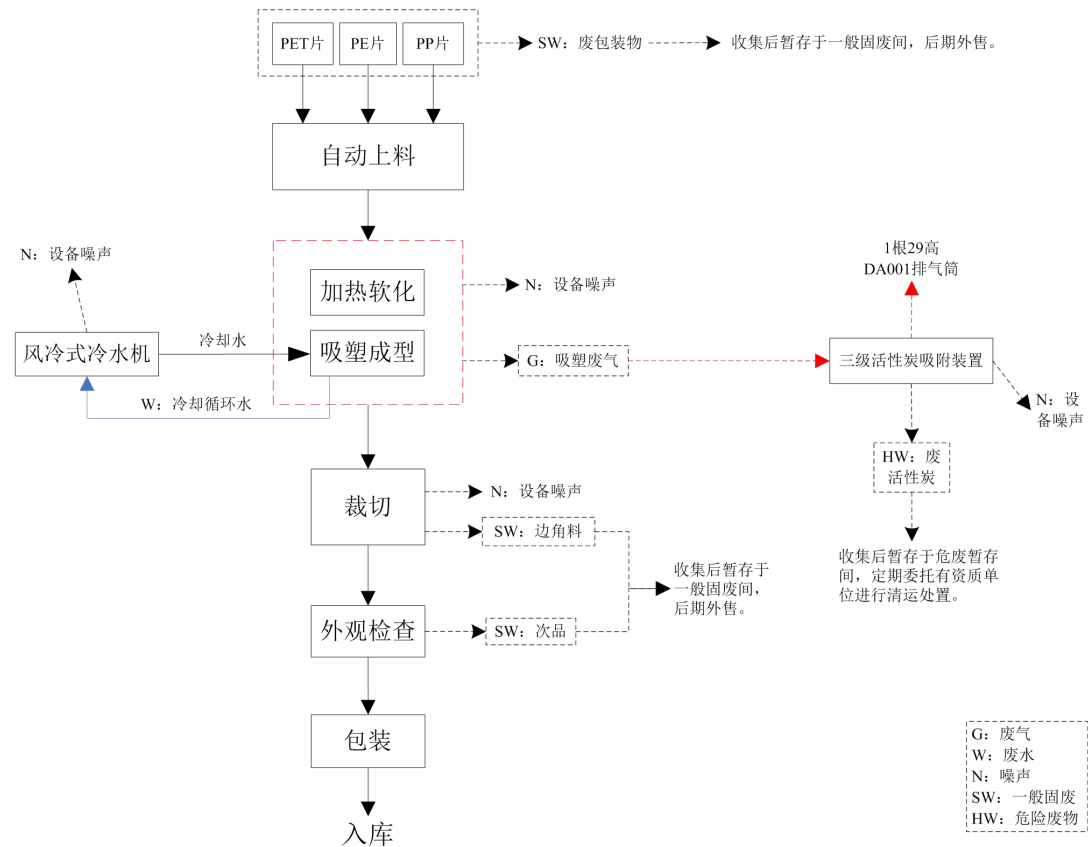
图 2-3 本项目工艺流程及产污节点图 工艺流程及产污环节简述：
