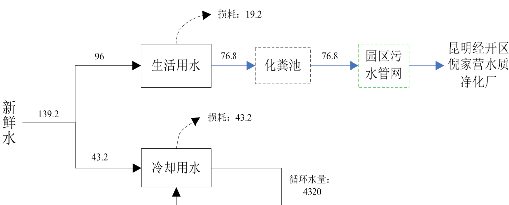
图 2-1 本项目建成后水量平衡图（单位：m³/a）
