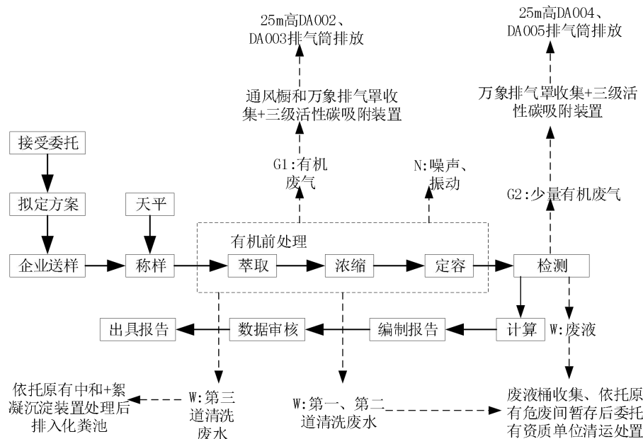
图 2-3 项目运营期有机实验工艺流程及产污环节图
