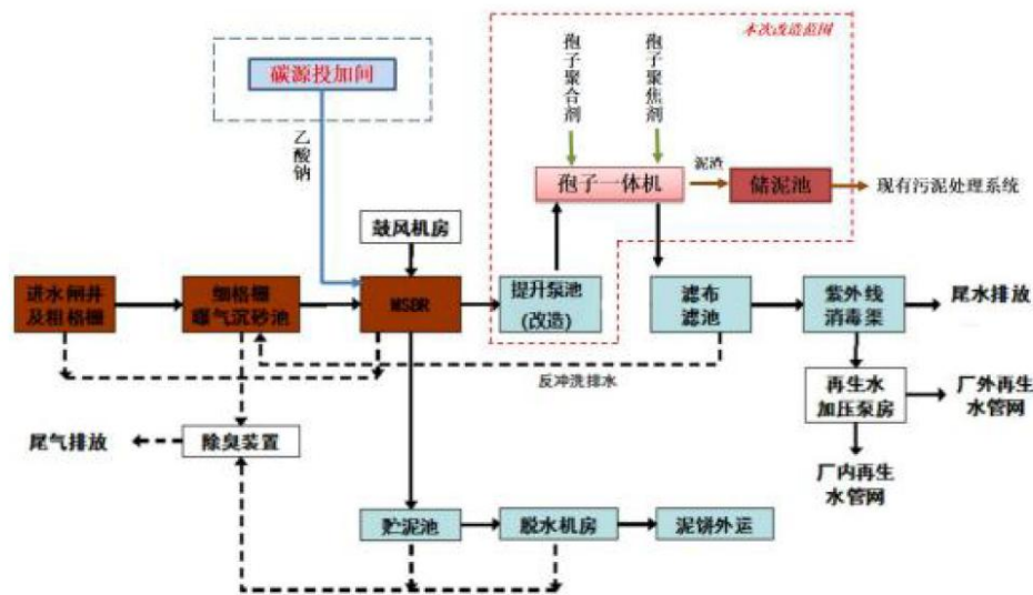
图 4-1 昆明第十二水质净化厂工艺流程图
