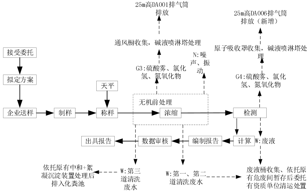
图 2-4 项目运营期无机实验工艺流程及产污环节图
