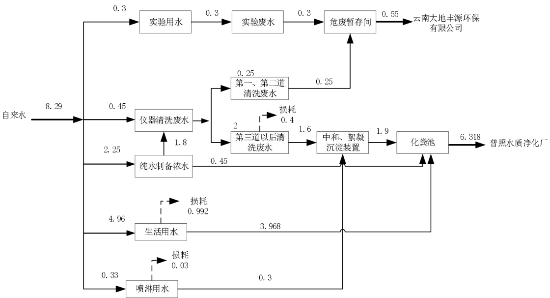
图 2-2 扩建完成后水平衡图 单位：m³/d
