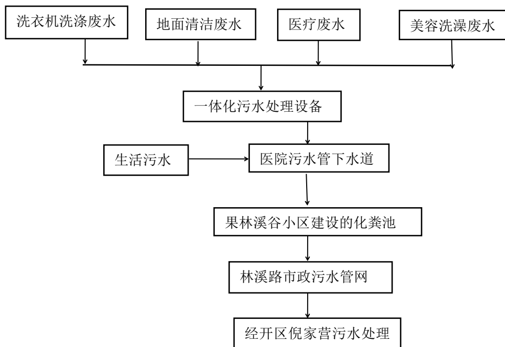
图 4-2 医院污水收集、处理流程
