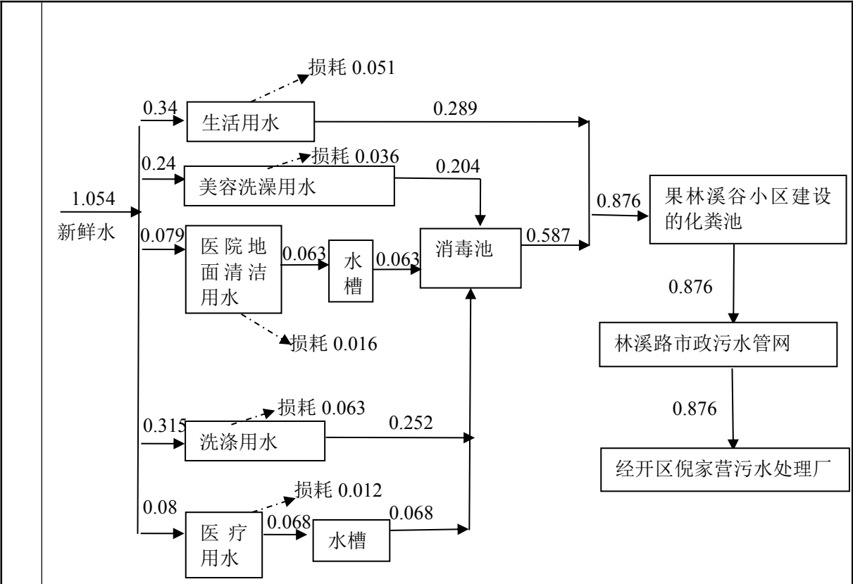
图 2-3 医院现有项目水平衡
