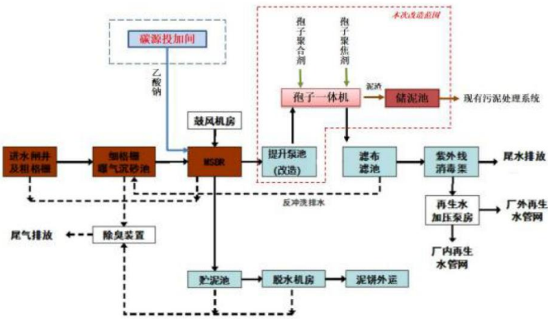
图 4-1 昆明第十二水质净化厂工艺流程图
